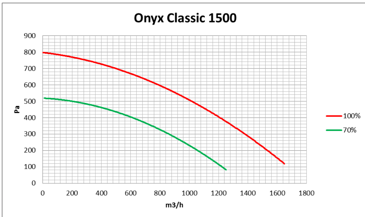
Rys 3. Wykresy wydajności centrali Onyx Classic 1500
