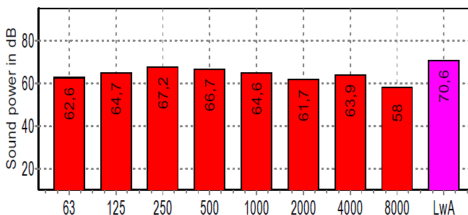
Rys 5. Charakterystyka wentylatora 1500+
