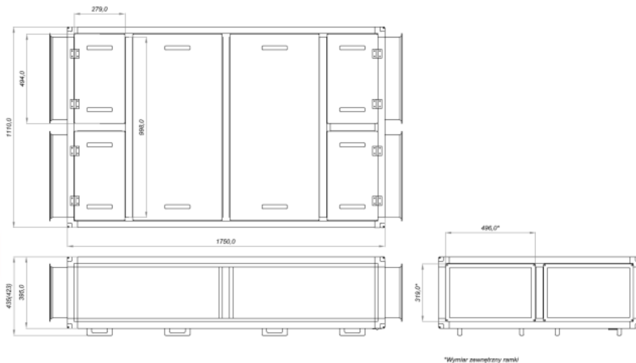
Rys 1. Wymiary zewnętrzne centrali wentylacyjnej OnyX Classic 1500
