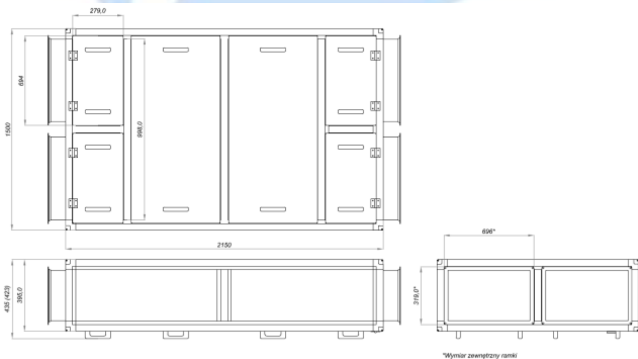
Rys 2. Wymiary zewnętrzne centrali wentylacyjnej OnyX Classic 1500+
