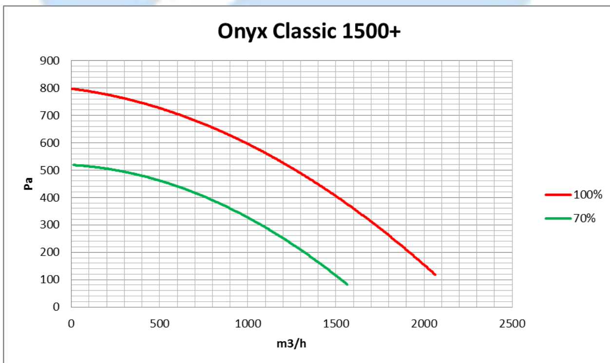
Rys 4. Wykresy wydajności centrali Onyx Classic 1500+
