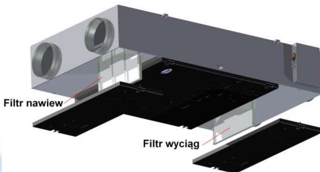
Rys 9. Wymiana filtrów centrali wentylacyjnej
