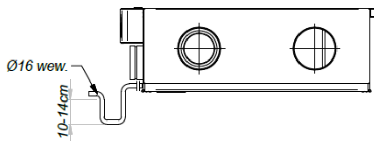
Rys 6. Układ odprowadzania kondensatu z centrali wentylacyjnej
