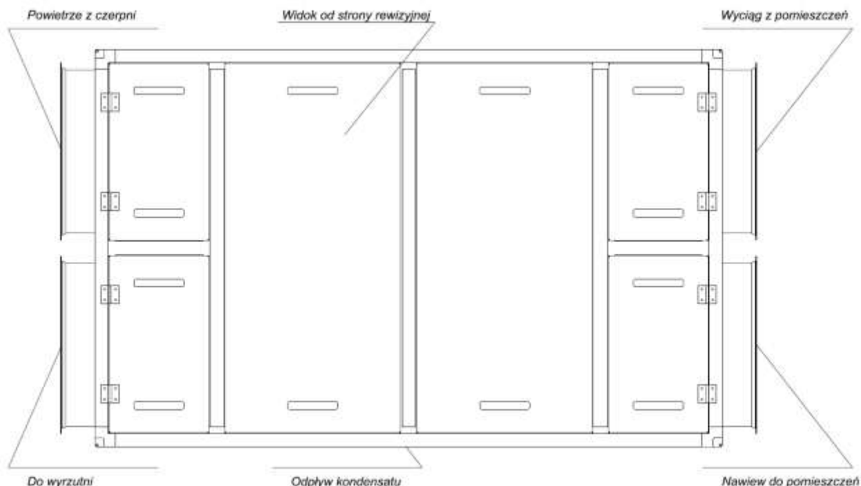
Rys 7. Rozmieszczenie króćców centrali wentylacyjnej OnyX Classic 1500 oraz OnyX Classic 1500+
